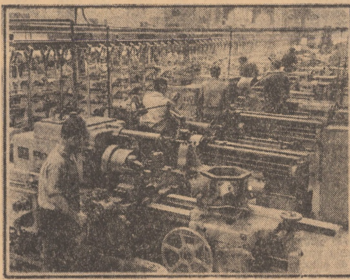
Una din cele trei linii de prelucrare a arborilor cardanici, cu o lungime totală de aproximativ 300 metri
