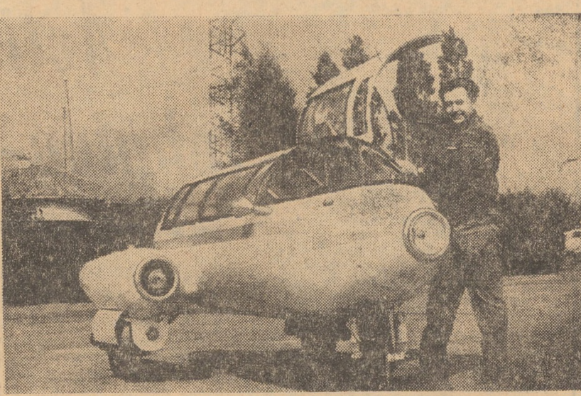
R.P. BULGARIA. În foto: tehnicianul Evstatil Stavev, din Varna care a obținut, de curînd, din partea autorităților respective, permisiunea de a circula pe drumurile publice cu această mașină, avînd forma unui avion, construită de el
