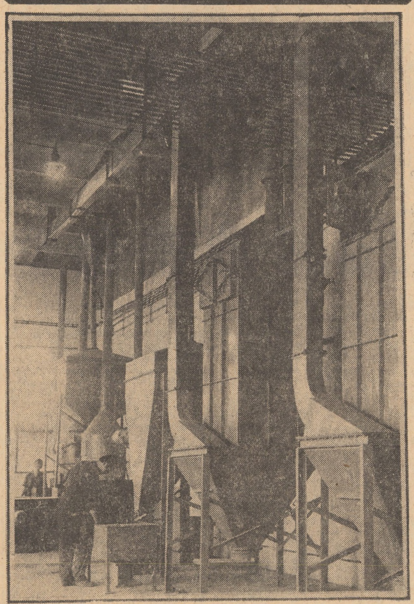
Instalația de preparare a nisipului pentru agregatele de formare în coji de beton din atelierul anexă a turnătoriei întreprinderii AMET Sibiu
