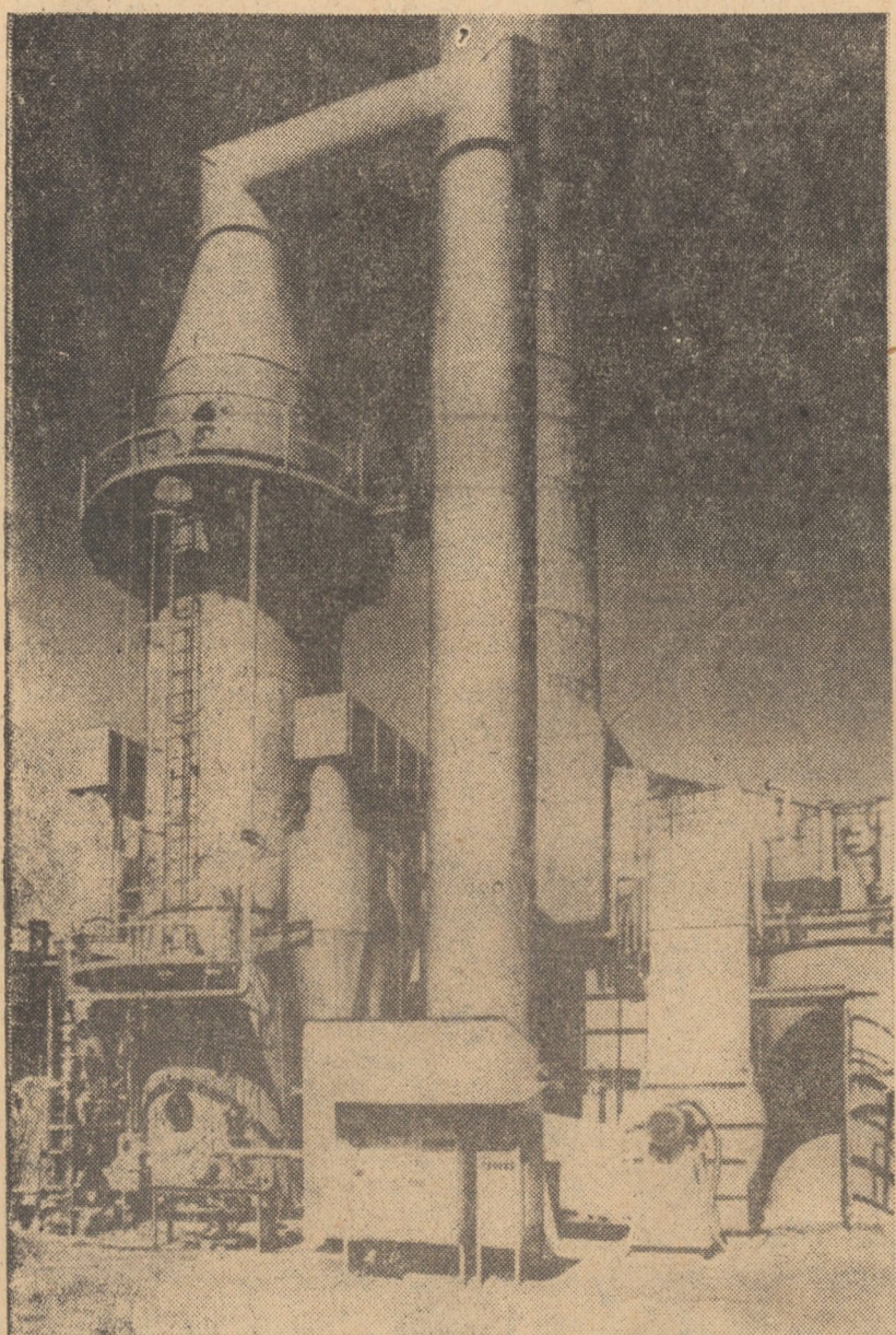
JAPONIA. În Japonia a fost realizat un proces de desulfurizare a deșeurilor de gaze, care recuperează semi-produse sub formă de particule uscate și nu emană nici un fel de poluanți secundari. Cu ajutorul acestei noi metode, gazele fluide și soluțiile alcaline sînt amestecate într-un turn de reacție special și produsele acestei reacții, în special sulfurile de sodiu, sînt transformate într-o pudră uscată. În foto: instalațiile de desulfurizare
