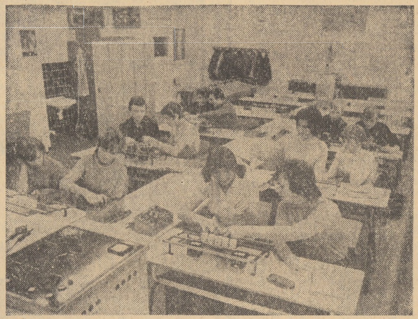
R.D. GERMANĂ. Peste 1400 de elevi între 13-16 ani participă la cursuri tehnice la uzina de vehicule și arme de vîntoare „Ernst Thälmann” din Suhl. Elevii mai mari ai școlilor tehnice învață cum să aplice cunoștințele acumulate în tehnica lemnului, metalelor și materialelor plastice.
