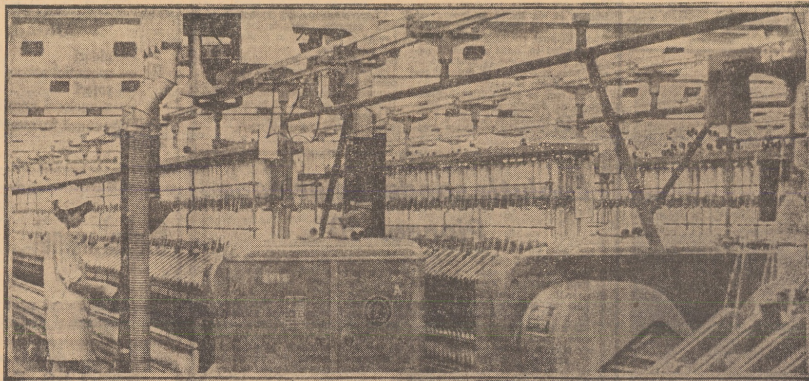
Mașina cu inele în filatura fabricii „Furul roșu”, Tîlmacia
