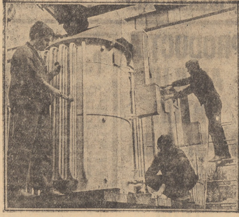
I.R.E. Sibiu — Două dintre bobinele de stingere de 20 kV — 50 A...
