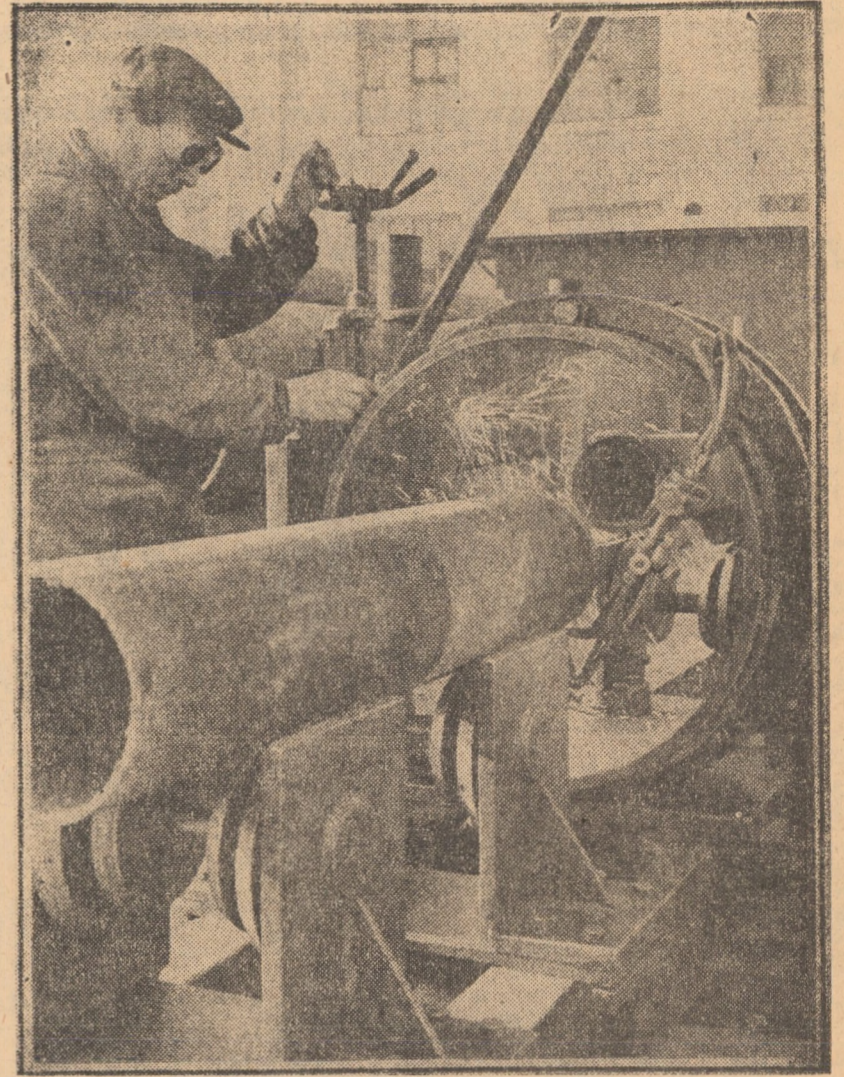
Dispozitiv pentru tăiat și sanie- nat țevi prin tăiere oxii-acetilenică — realizat prin autoutilare la Uzina mecanică gaz metan
