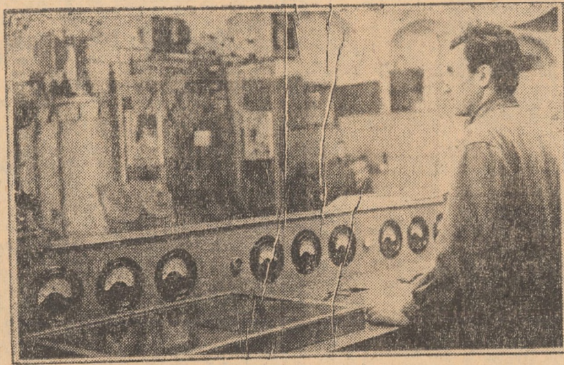
La standul de probe pentru verificarea calității reparațiilor executate la I.R.E. Sibiu, secția reparat mașini electrice, maistrul Dumitru Radu verifică — la panoul de comandă — rezistența de izolație la un transformator
