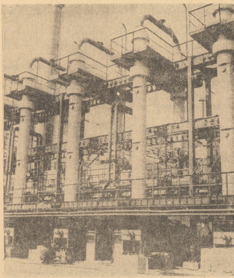
R.P. POLONĂ. Aspect de pe șantierul noii fabrici de negru de fum, aflată în construcție în imediata apropiere a realizării de petrol de la Maslovojevodul Rzeszon. Negrul de fum realizat aici, va fi folosit, în cea mai mare parte la fabricarea anvelopelor
