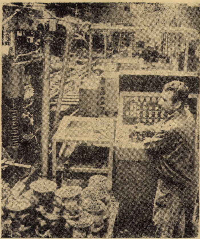
Linia de transfer automată de la I.P.A. Sibiu a fost concepută de specialiștii întreprinderii și confecționată în mare parte prin autototare
