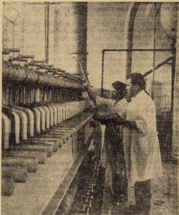
Întreprinderea de bere și amidon Sibiu, secția fierbere. Filtru — presă prin care trece întreaga cantitate de plămădă din care apoi se obține mustul de bere în funcție de sortimentul dorit. În fața utilajului: maistrul Cornel Coldea și operatora Ana Simion recoltînd o probă pentru analiza de laborator
