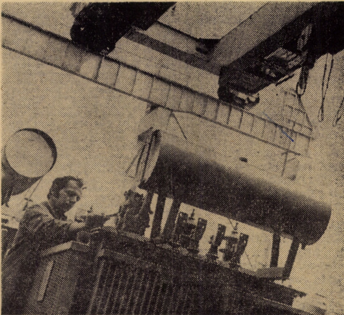
Electricianul Ștefan Birlea, efectuînd o ultimă verificare a bobinelor de stingere și a transformatoarelor de nul pe rampa de expediție a I. R. E. Sibiu Foto: FR. NUSS
