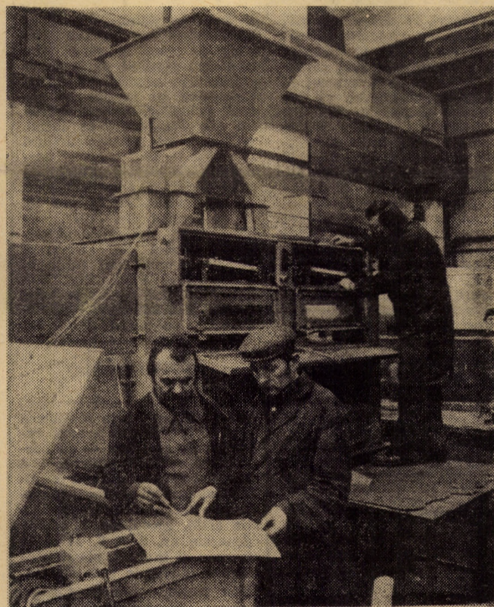
În atelierul unicat al întreprinderii „Balanța“ din Sibiu o nouă premieră: Bascula semiautomată pentru materiale granulare de 30 kg cu o capacitate de încăuire de 300 saci/oră, destinată industriei chimice. În anul 1980, aici se vor realiza un număr de 14 asemenea utilaje Foto: FRED NUSS
