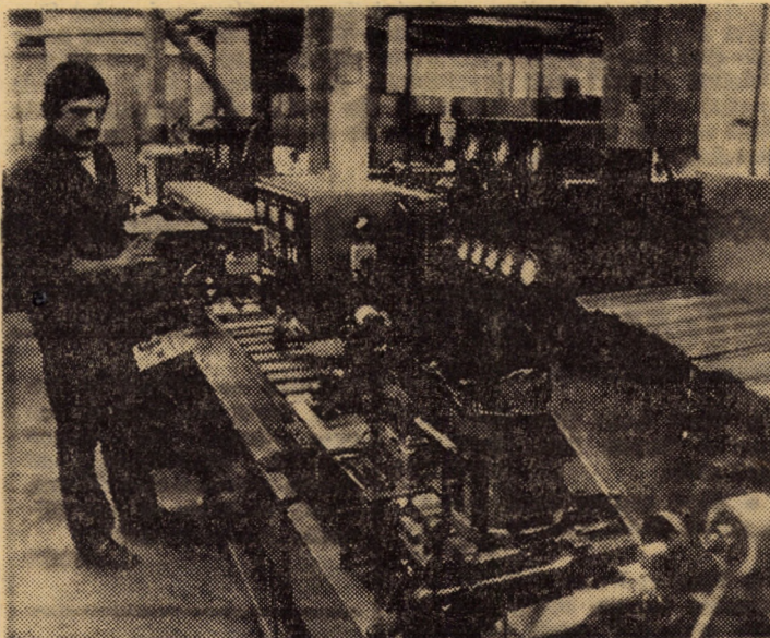
Utilajul din fotografie reprezintă o linie modernă, complet automatizată de fabricat creioane, realizînd o producție de cca 170 000 creioane într-un schimb, instalată într-o nouă hală de producție la I.P.L. Sibiu
