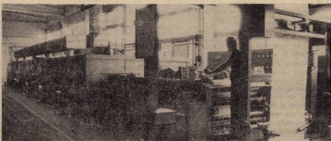
Cu ajutorul unui utilaj de mari proporții din secția finisaj a întreprinderii „Tirnavă” Mediaș se asigură termofixarea țesăturilor cu conținut de 50 la sută fire din poliester. Astfel contracția la spălătul casnic al acestor produse se menține sub 2 la sută Foto: FRED NUSS
