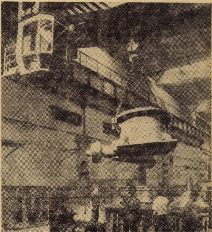
Descărcarea unui granulator giratoric la bancul de probă tehnologică în secția mecanică II a întreprinderii „Independența” Sibiu. Foto: Fred NUSS
