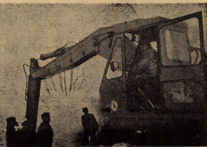
Într-un timp record (48 ore) și în condiții dificile, constructorii de la I.C.M.J. Sibiu au executat în zona Cîrța una dintre cele mai grele lucrări de pe traseul conductei de alimentare cu apă a orașului Agnita — subtraversarea geselei E 15 A
