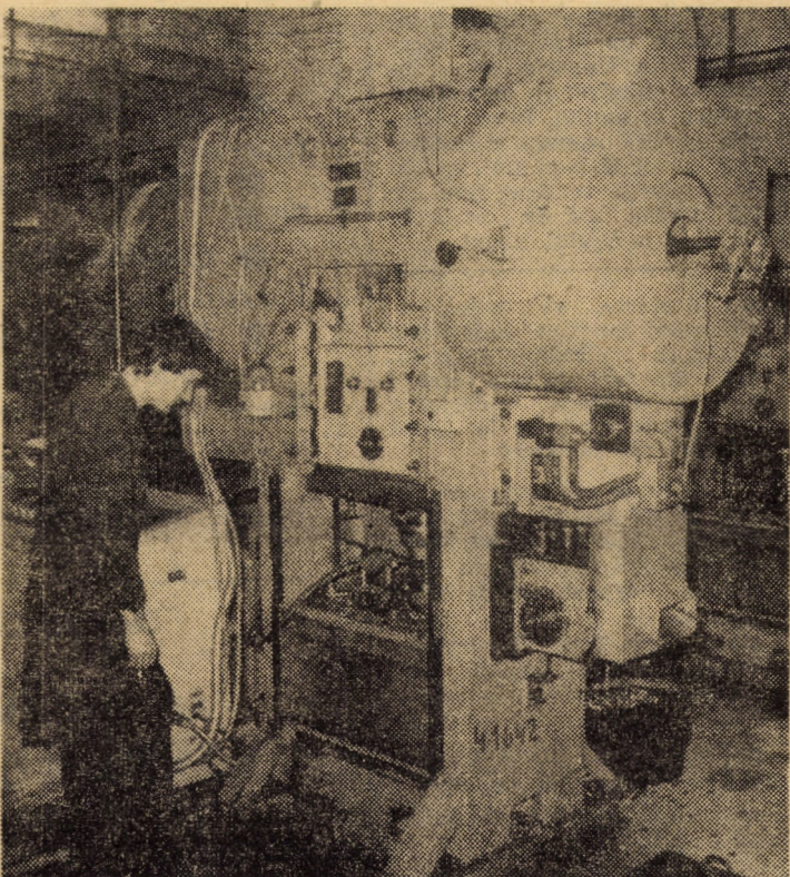
Întreprinderea mecanică Mediaș, sectorul II. În atelierul saibe elastice și nituri speciale, cu ajutorul preselor de ștanțare rapidă P.M.R.S. (produse de Întreprinderea mecanică din Sibiu), se obțin o serie de produse de mici dimensiuni, destinate autoturismelor „Dacia” și „Oltcit”. Foto: Fred NUSS
