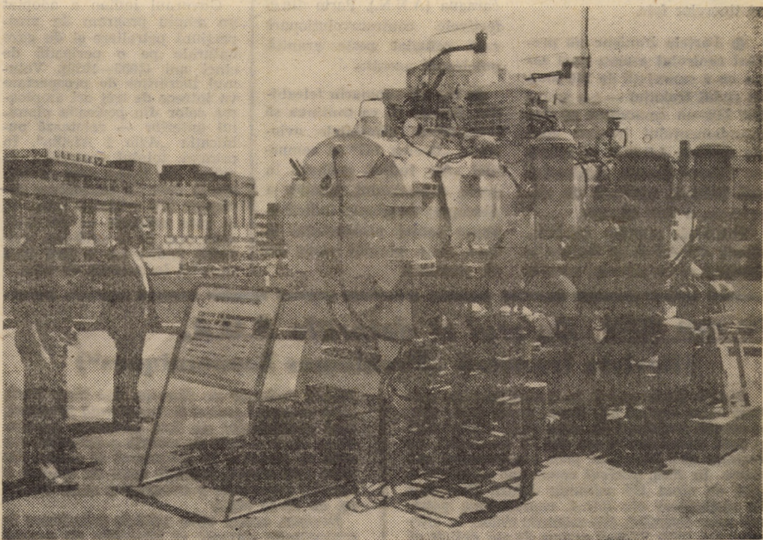
Unul din exponatele care a stîrnit un interes deosebit la „Expoziția realizărilor economico-sociale ale județului Sibiu” a fost și „Cuptorul pentru tratament termic în vid”, pe care vi-l redăm imaginea de mai sus
