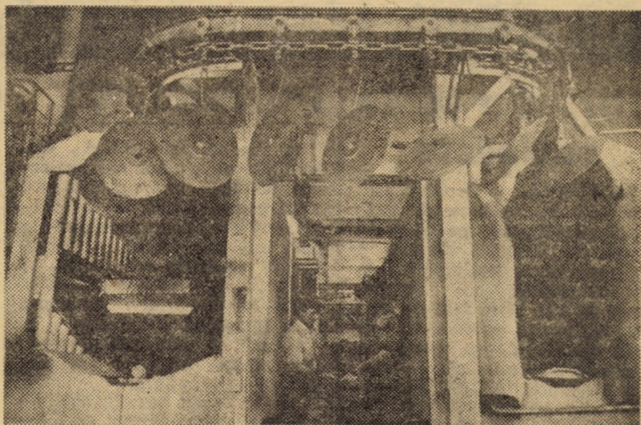
I.M.A.I.A. Sibiu. Linie automată de vopsit piese de schimb prin imersie, aflată în probe tehnologice Foto: Fred NUSS
