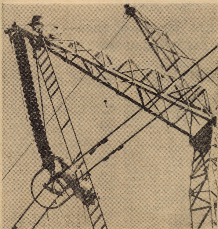
Secvență de lucru pe magistralele de transport al energiei electrice. Stilpi metalici, izolatoare, conductorii de înaltă tensiune și... oameni de mare curaj și profesionalism Foto: Horst BUCHFELNER
