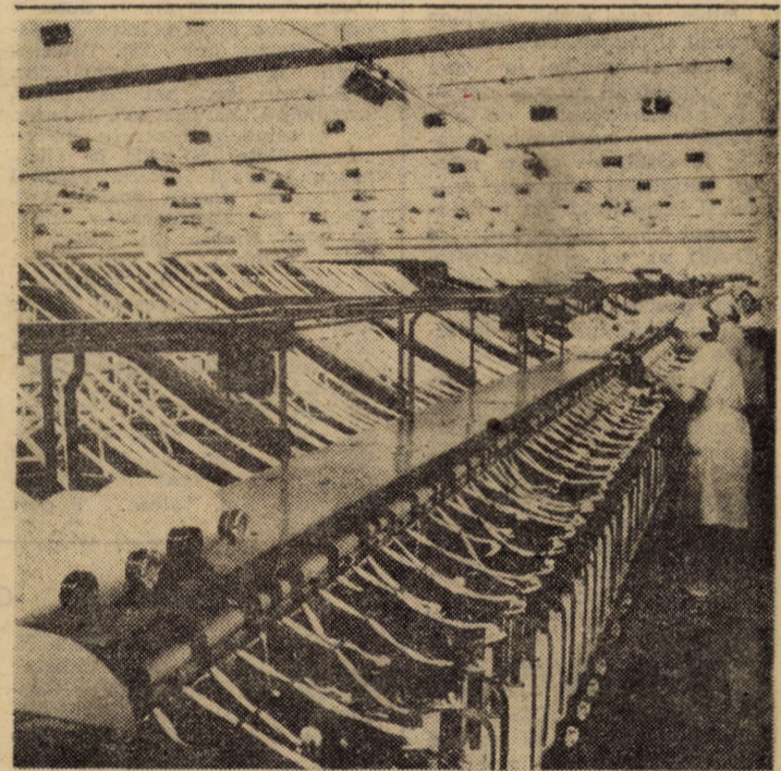
În imagine vă prezentăm grupul mașinilor de inele din secția filatură a întreprinderii „Firul roșu Tălmaciu” Foto: Fred NUSS
