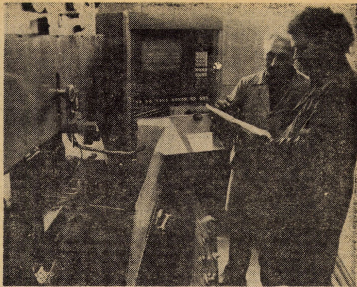
Întreprinderea de relee Mediaș, secția sculărie. S.D.V.-urile cu grad înalt de complexitate, necesare procesului de producție, sînt obținute cu ajutorul unor utilaje cu comandă program. În fotografie: șeful de atelier Tiberiu Bokor și operatorul Nicolae Popa urmărind programul de desfășurare a operațiilor de prelucrare la o mașină de prelucrat prin electroeroziune cu fir
