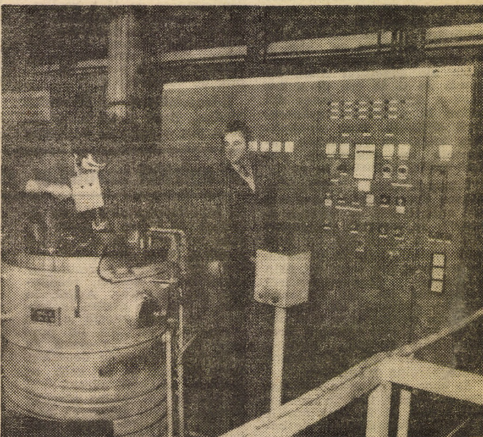
Întreprinderea Mecanica Sibiu. Procedul de tratare termică cu ajutorul instalației de ioniturare (în fotografie) se aplică pieselor de mare complexitate, supuse la uzură intensă Foto: Fred NUSS
