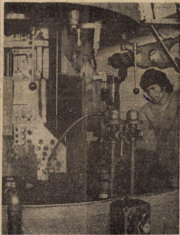
Prelucrarea prin așchiere a produselor la un strung semiautomat cu 6 axe verticale la I.M.A. Sibiu Foto: Fred NUSS
