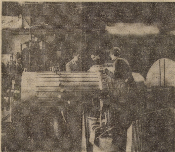
Rebobinarea unui transformator de putere în cadrul secției de utilaje, confecționat și reparat echipament energetic de la I.E.I.R.I.E.D.E.E.T. Sibiu
